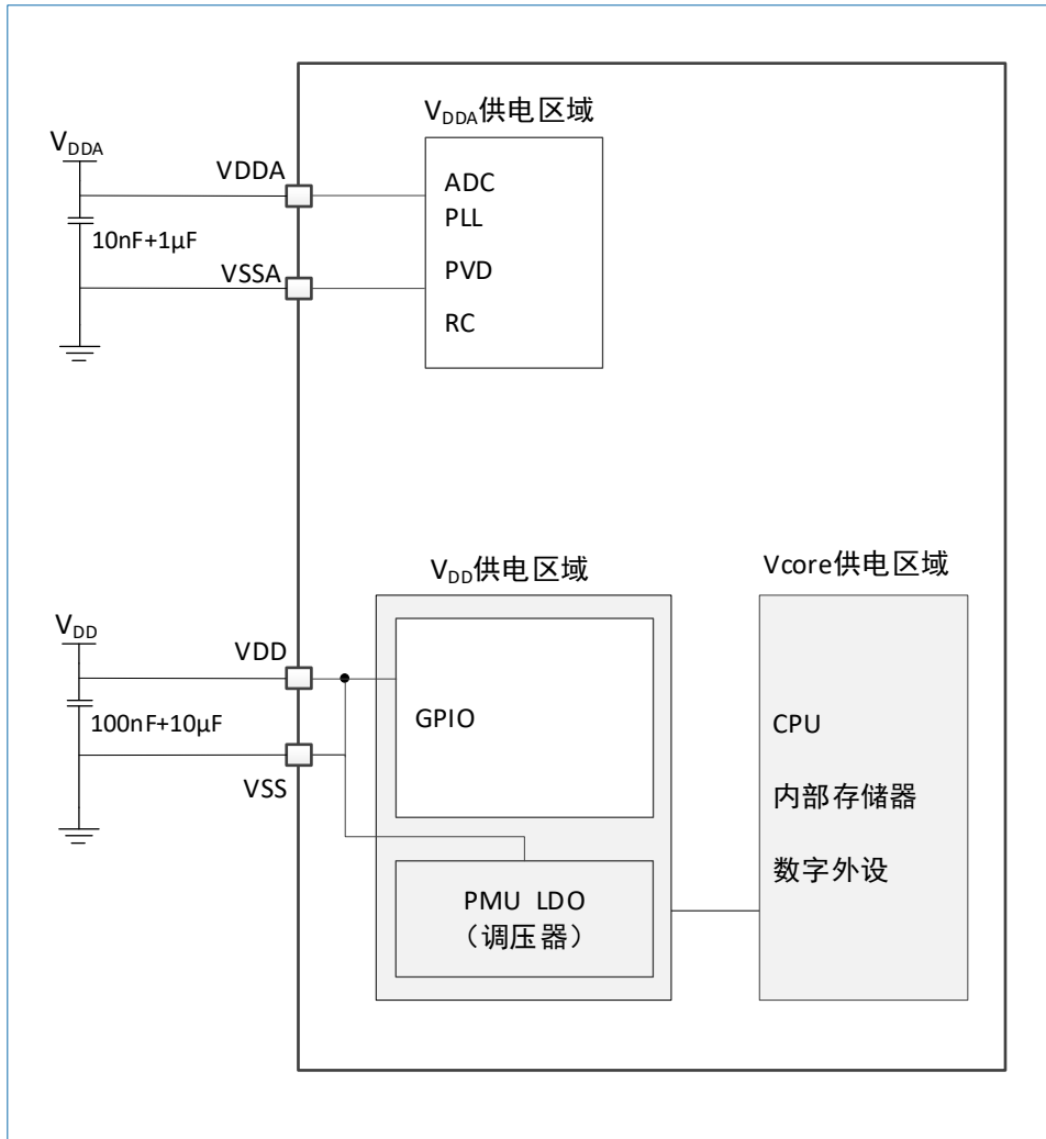
图 5-1 电源框图
