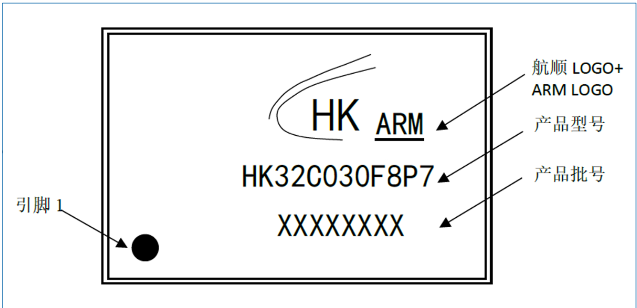
图 7-11 TSSOP20 丝印示例 (HK32C030F8P7)
