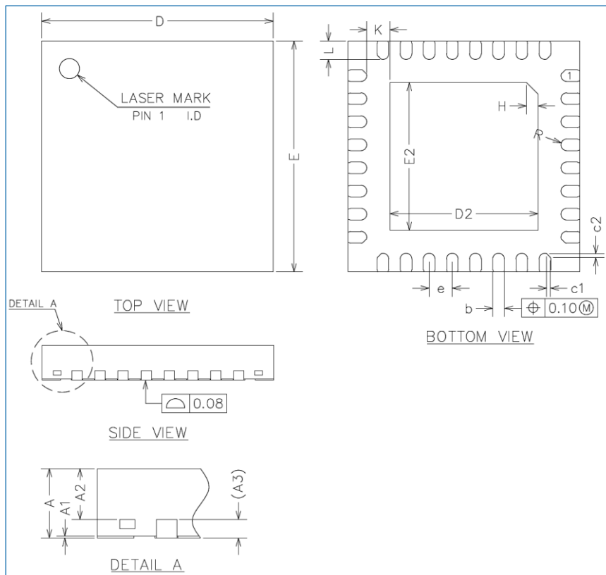
图 7-3 QFN32 封装尺寸图
