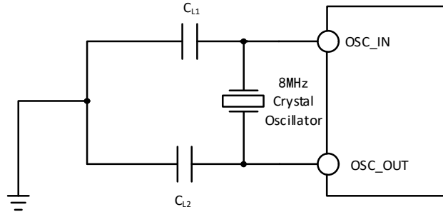
图 3-5 外接 8M 晶体典型电路
