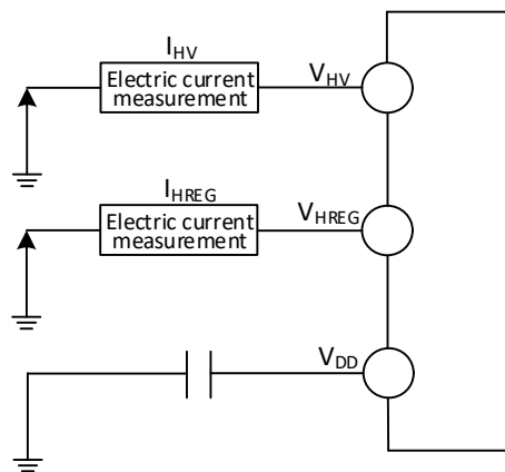
图 3-2-2 CH32M103G8R6 电流消耗测量
