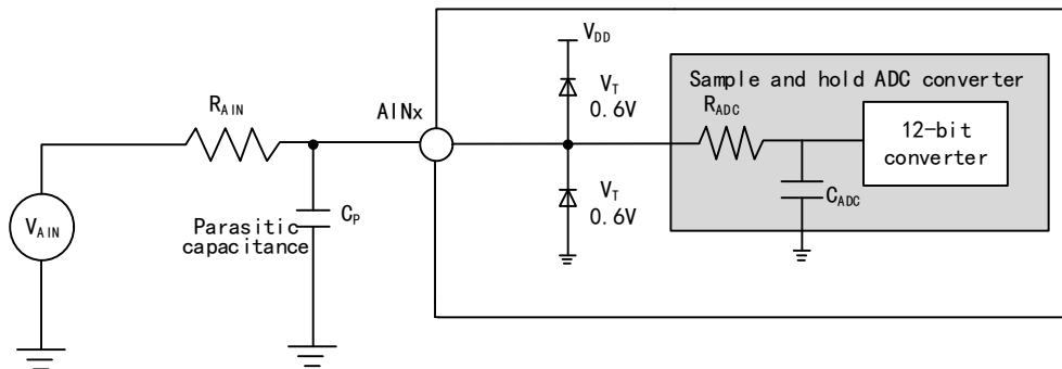
图 3-12 ADC 典型连接图
