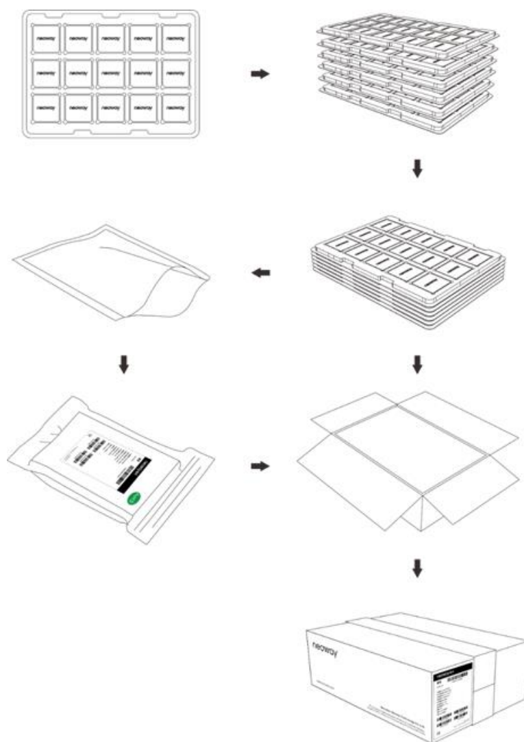
图 7-2 N723-EA 模组包装示意图
