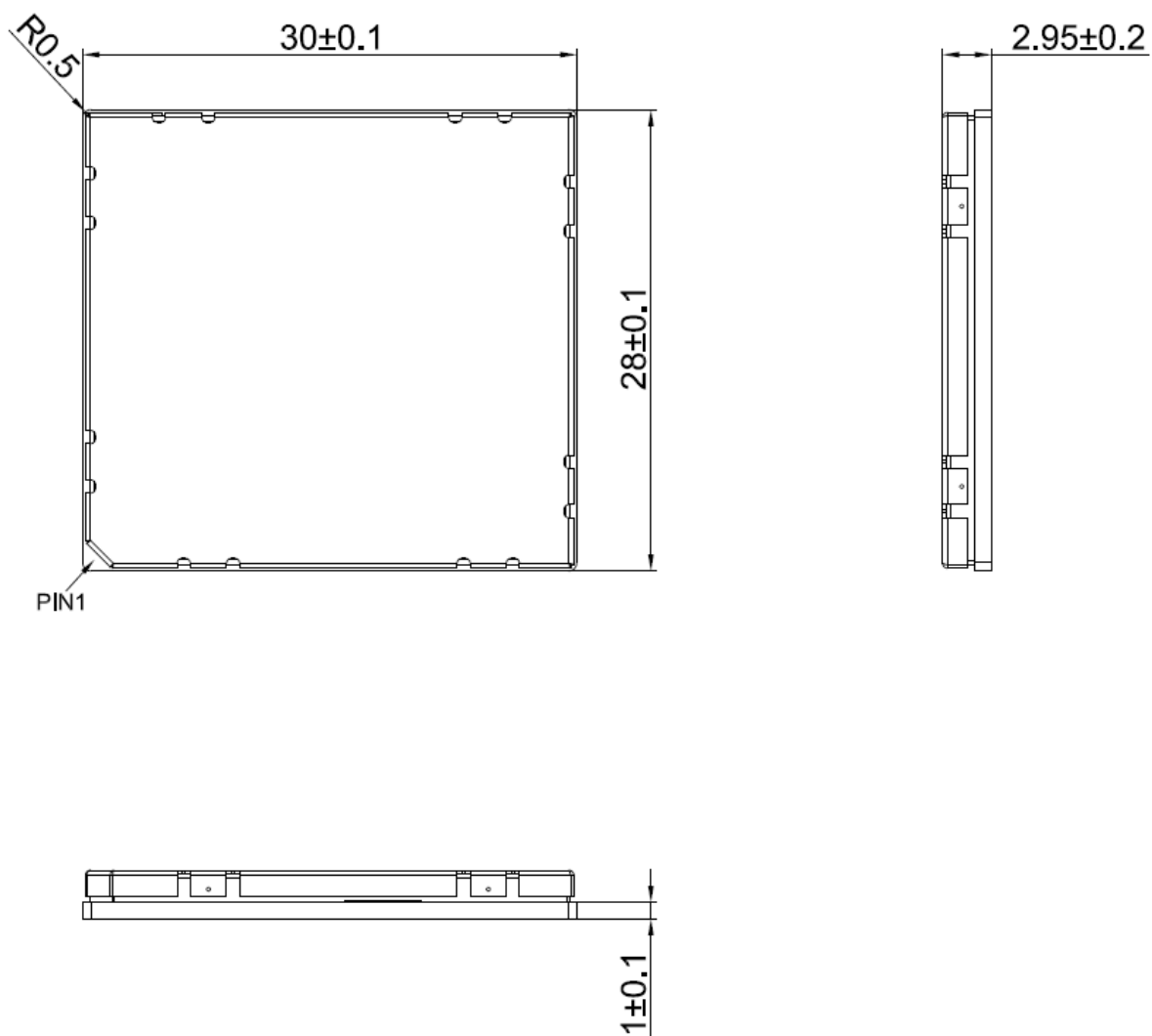
图 7-1 N723-EA 模组俯视图和侧视尺寸(单位: mm)
