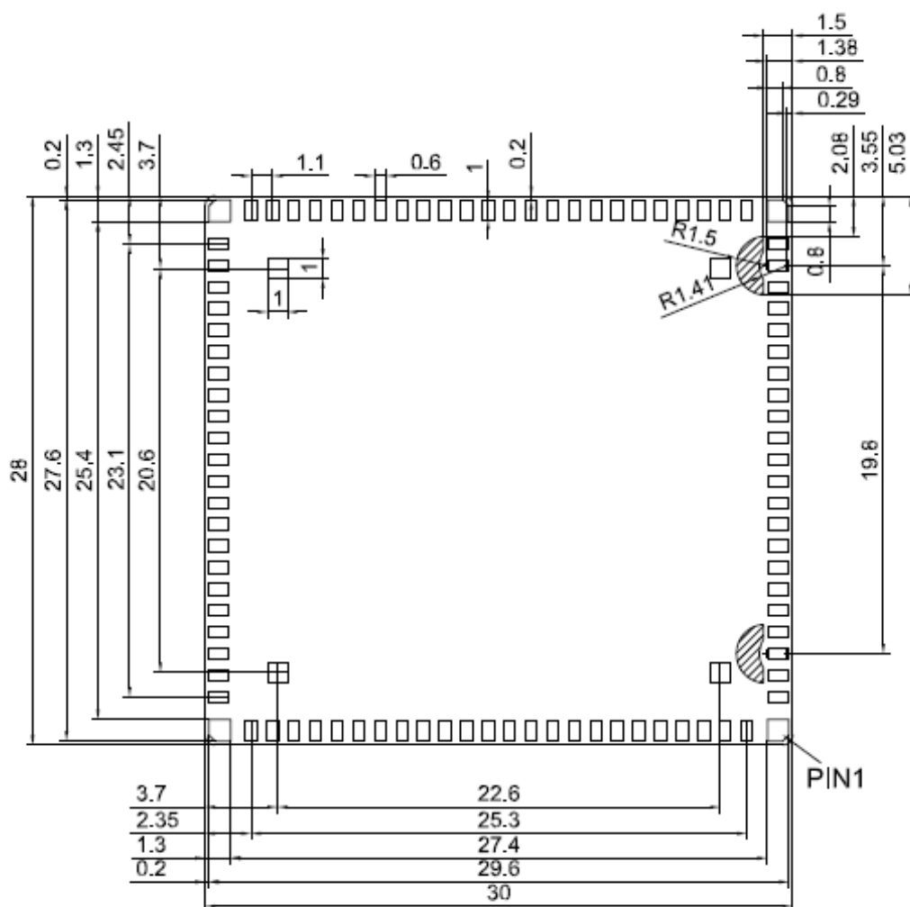
图 8-1 N723-EA 模组 PCB 封装底视图(单位: mm)
