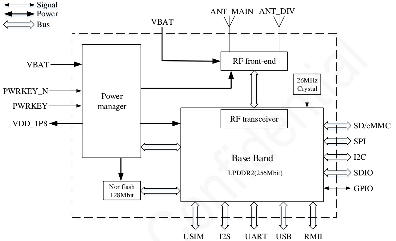
图 2-1 设计框图
