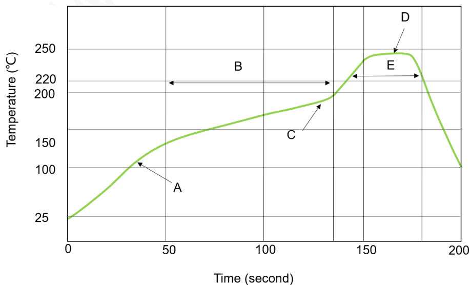
图 8-2 炉温曲线
