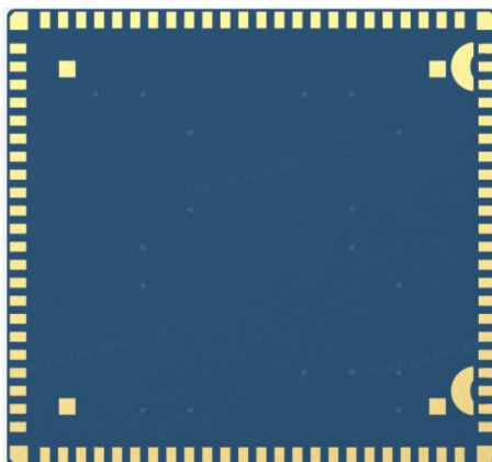
图 4-3 N723-EA 模组底视图
