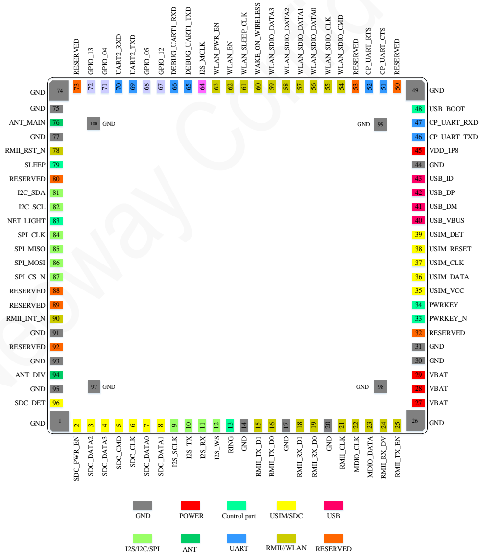
图 4-1 N723-EA 管脚定义 (Top View)
