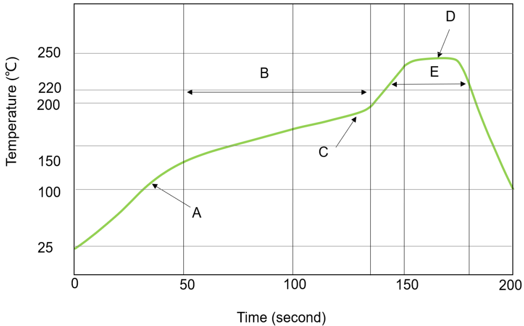
图 7-3 炉温曲线
