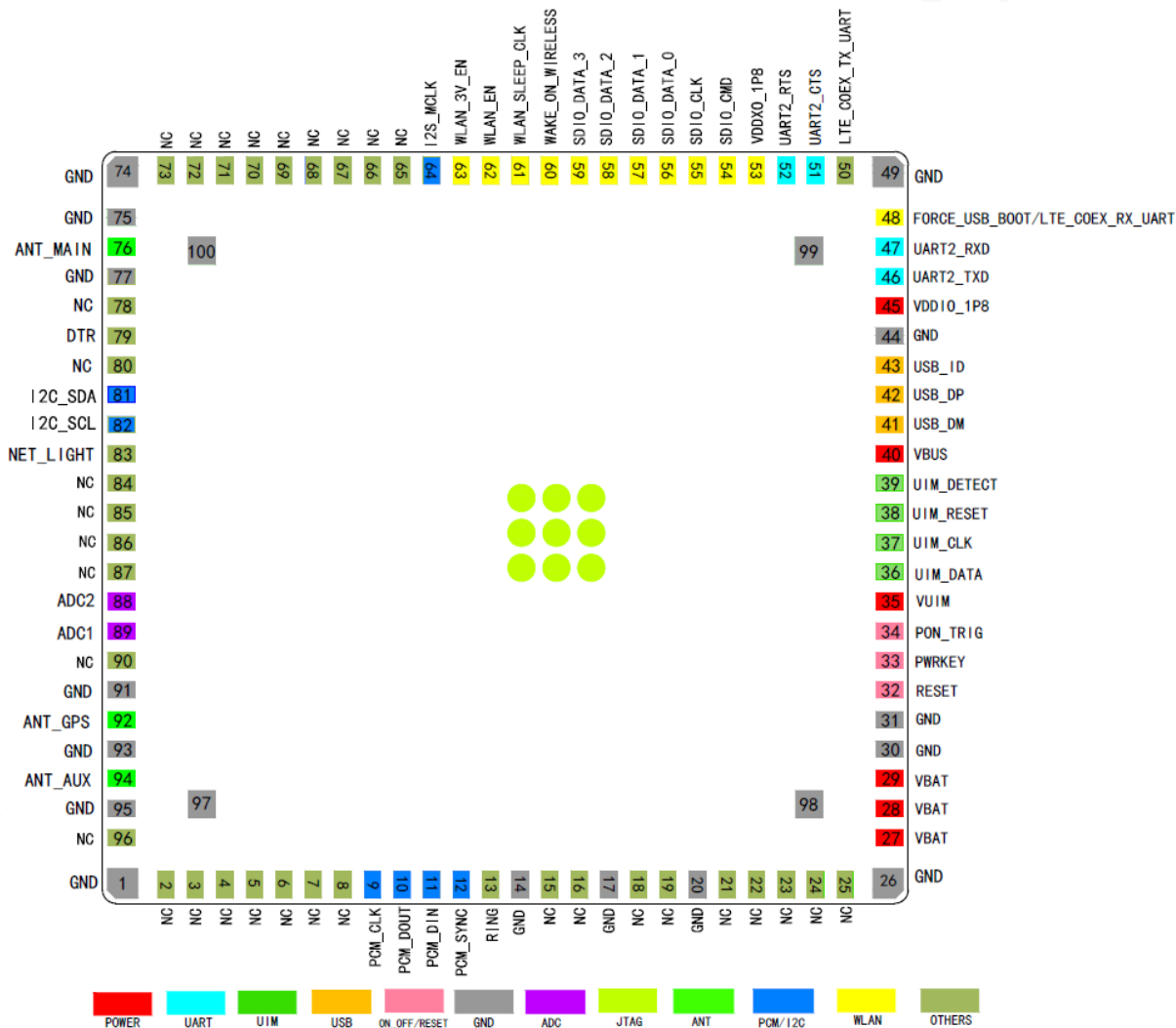
图 3-1 N720 模块管脚定义（Top View）
