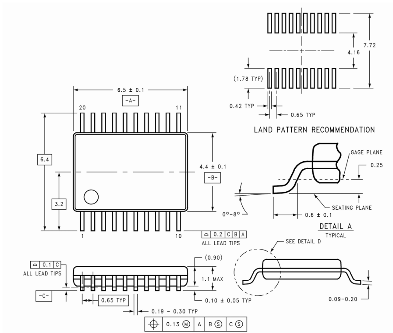
图10 TSSOP20 封装尺寸图
