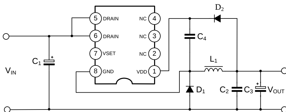
图1: 12V/0.3A输出时应用线路图
