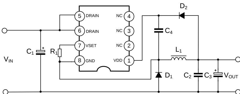
图1: 18V/0.3A输出时应用线路图
