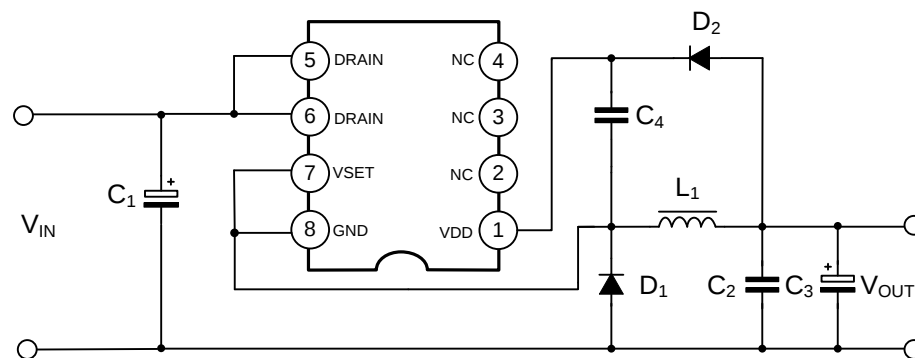
图1: 15V/0.3A输出时应用线路图
