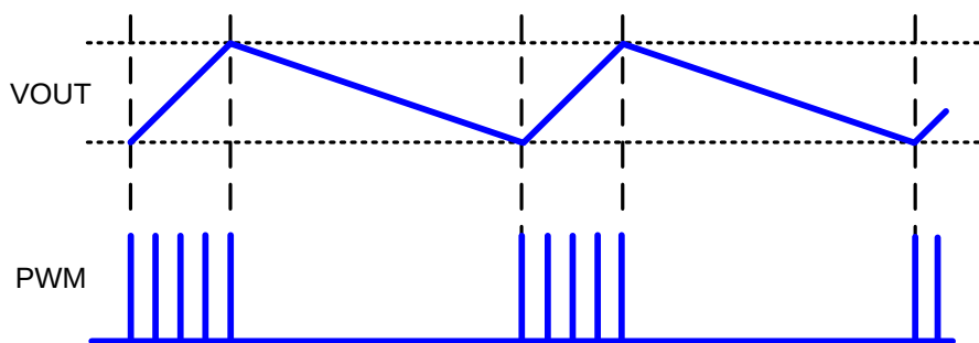
轻载打嗝波形
