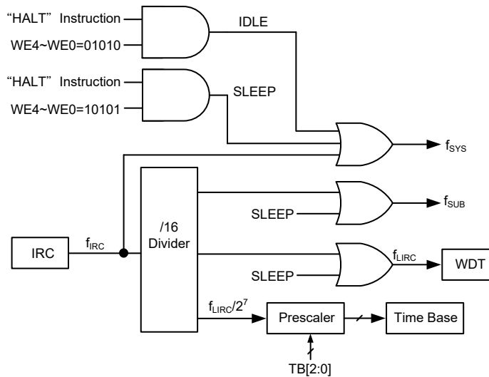
单片机时钟选项 – HT68F0012
