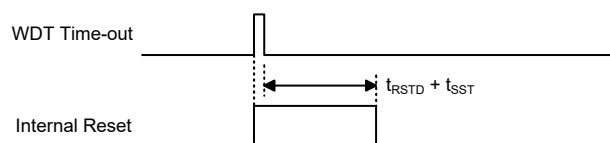
低速模式时看门狗溢出时序图
