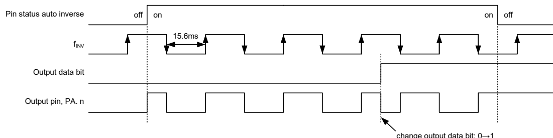
引脚状态自动反相功能时序图
