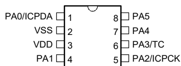
HT68F0017 8 SOP-A
