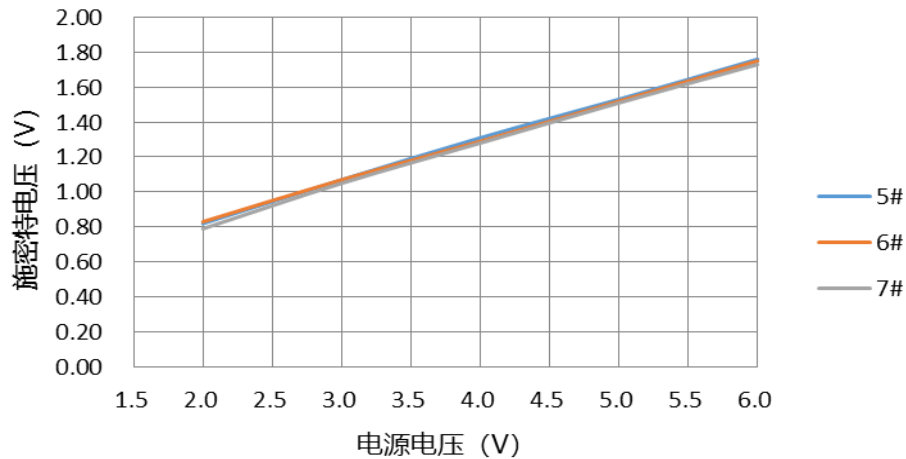
VIH电压VS电源电压@输入高@SMTEN=0
