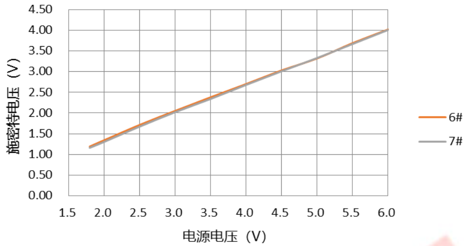
VIH电压VS电源电压@输入高@SMTVS配置2
