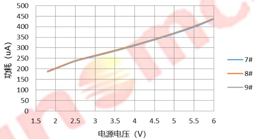
IDD功耗VS电源电压@FCPU=500KHz@HIRC
