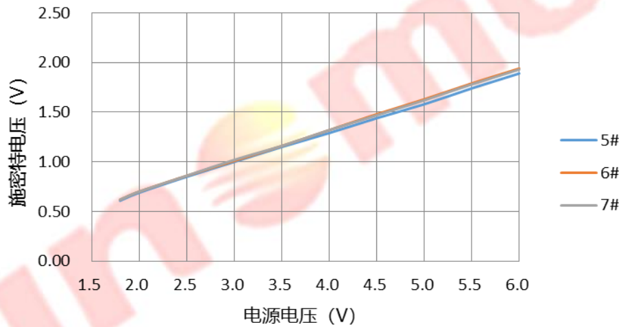
VIL电压VS电源电压@输入低@SMTVS配置2
