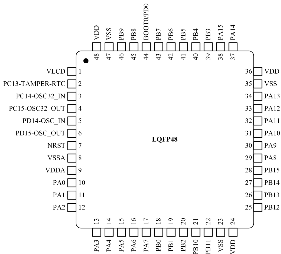
图 3-2 CM32M101A系列LQFP48引脚分布
