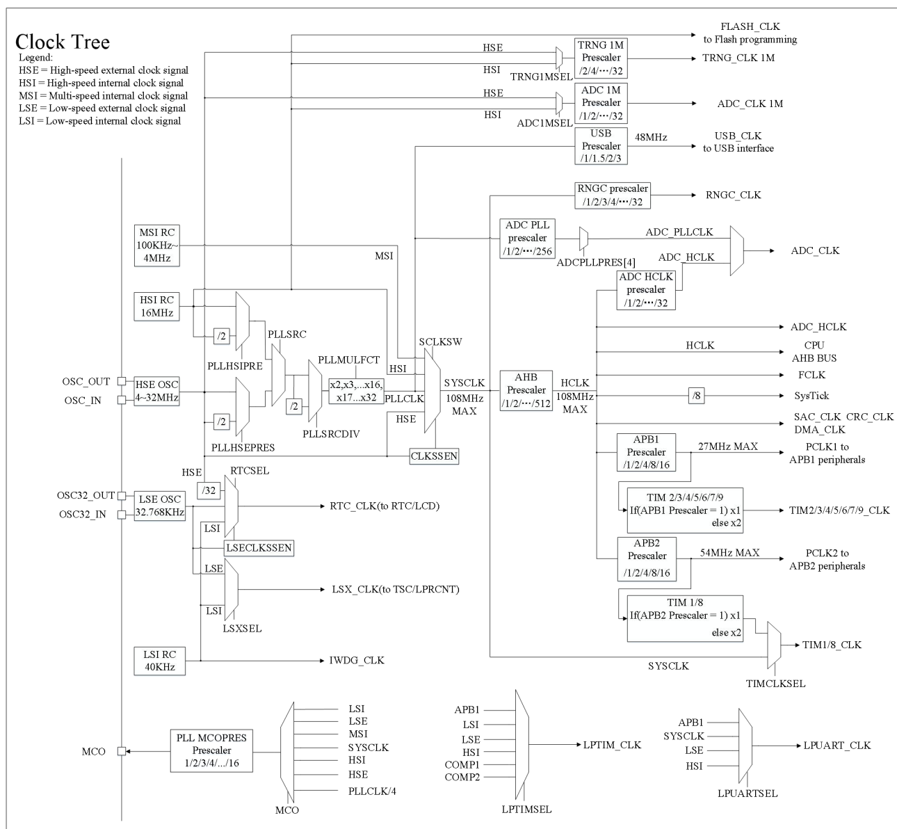
图 2-2 时钟树
