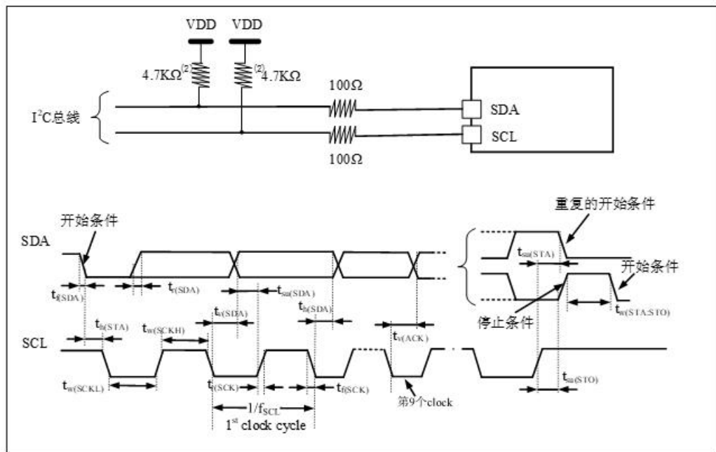
图 4-11 I 2 C总线交流波形和测量电路 (1)
