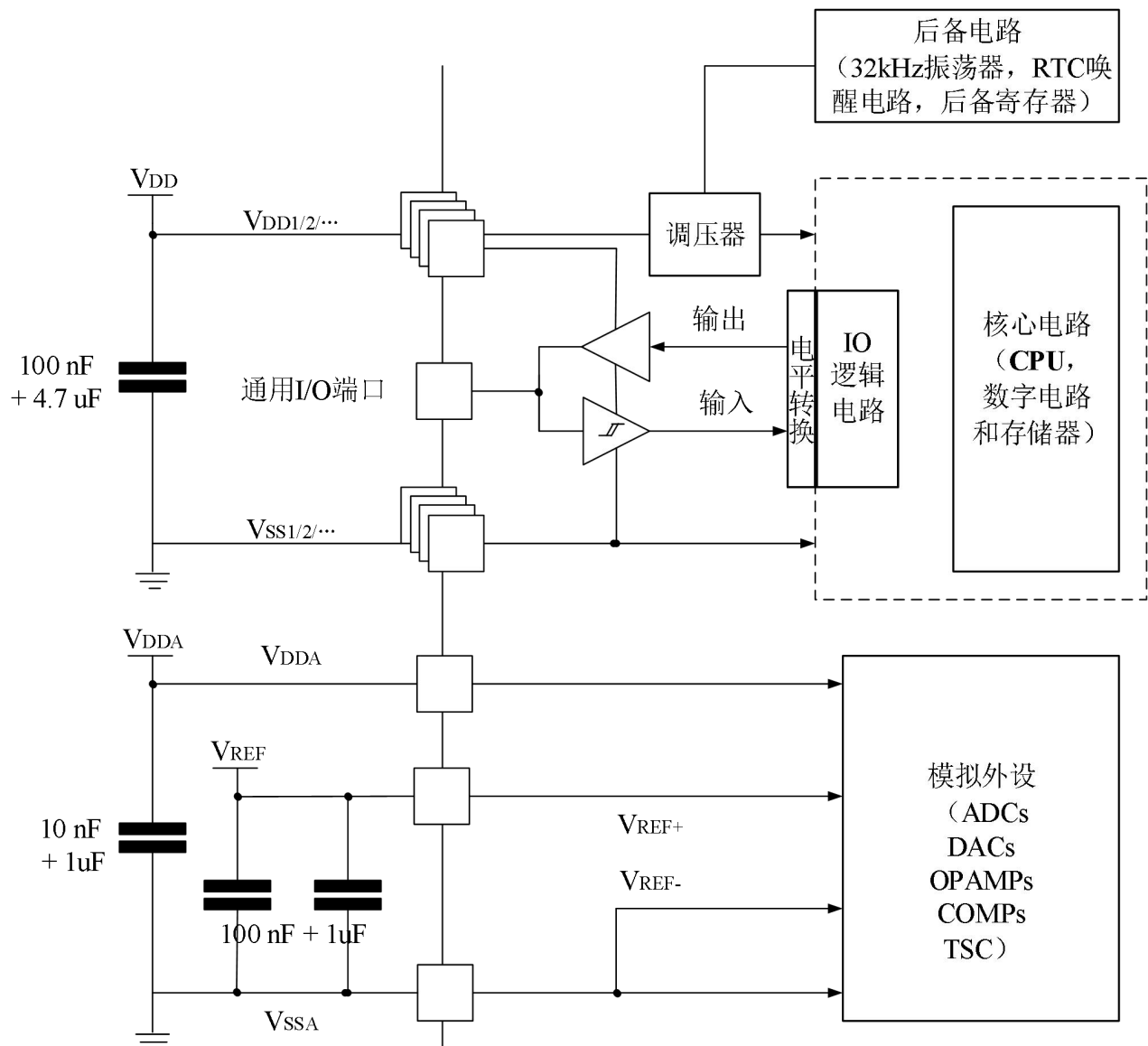
图 4-3 供电方案
