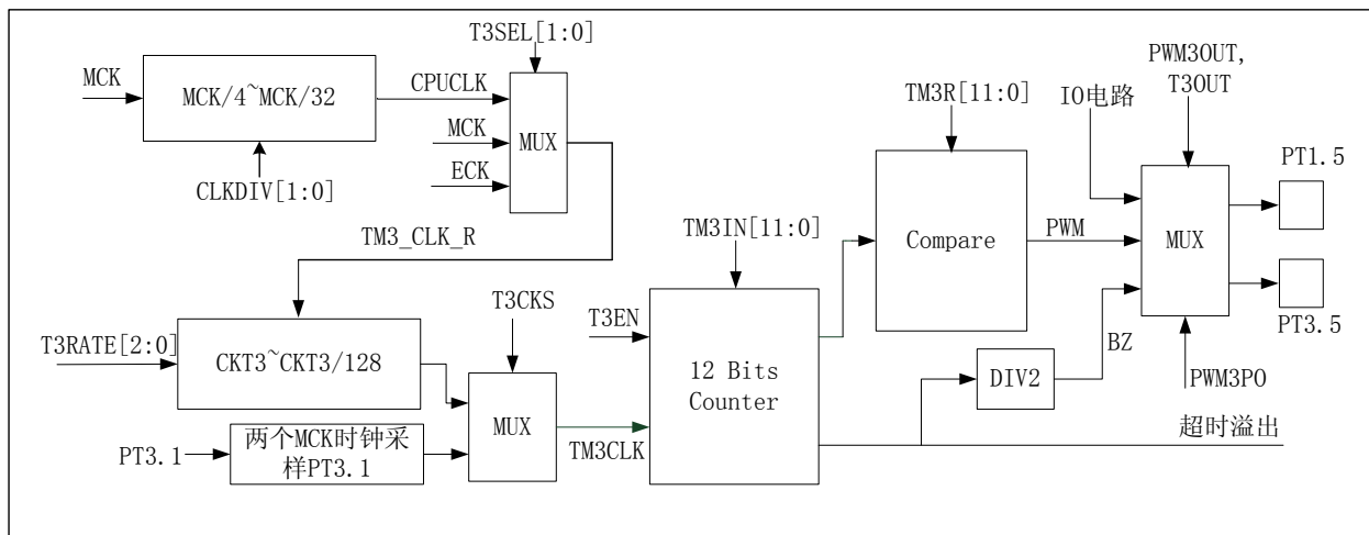
图17 定时/计数器3模块的功能框图
