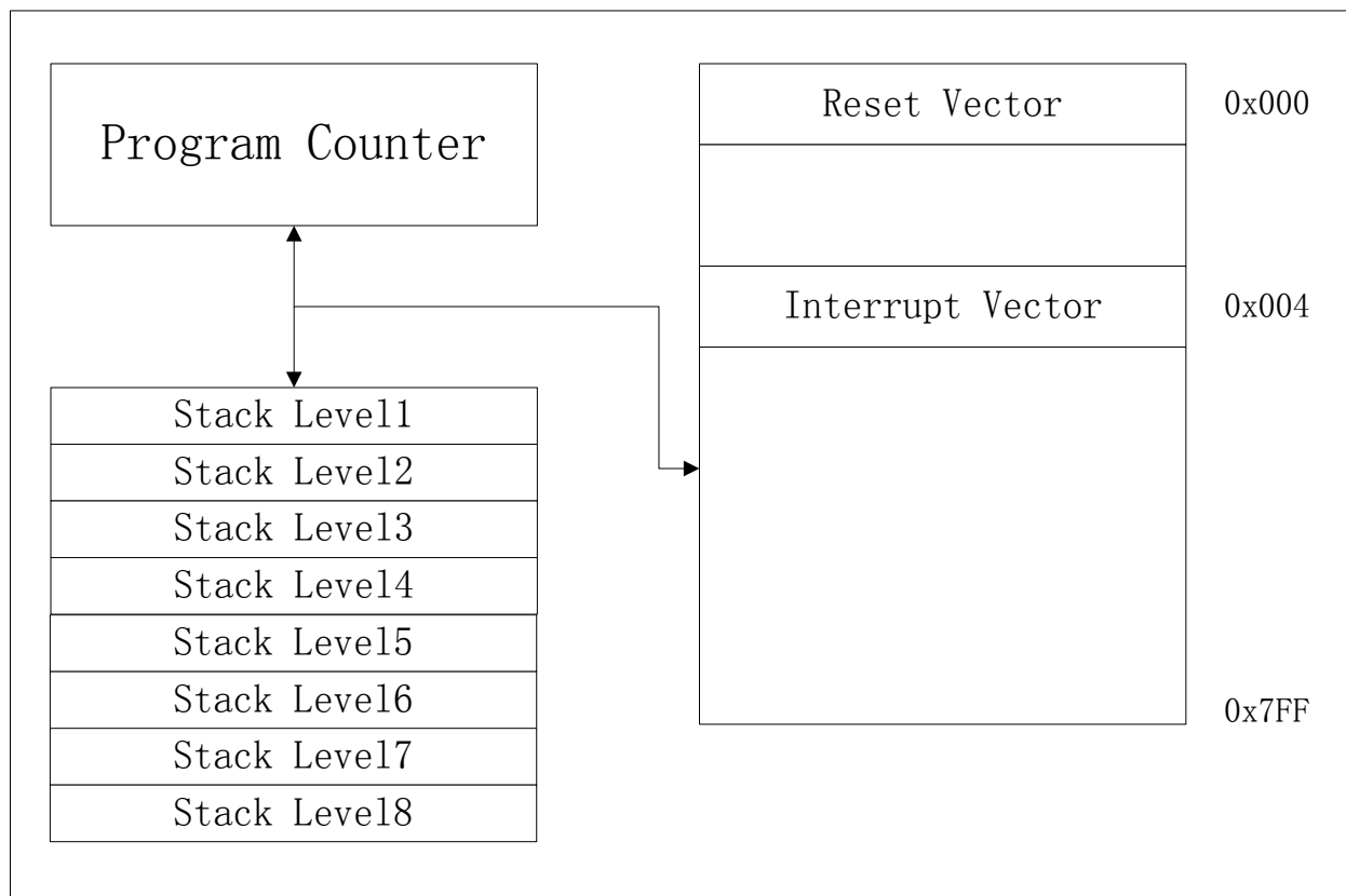
图5 程序存储器
