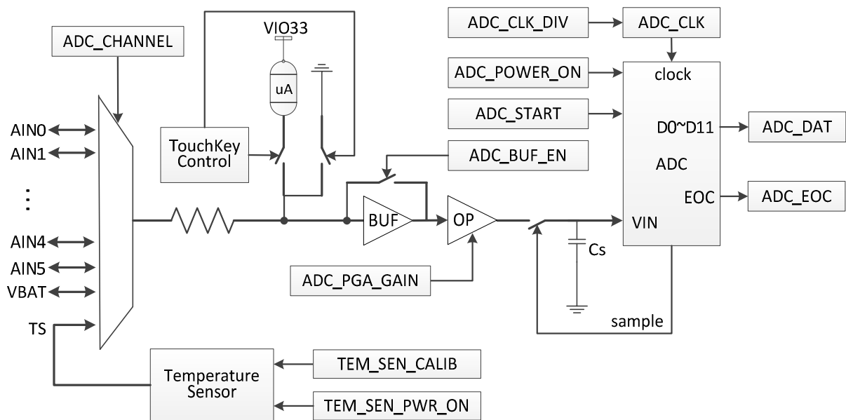
图 15-1 ADC 结构图
