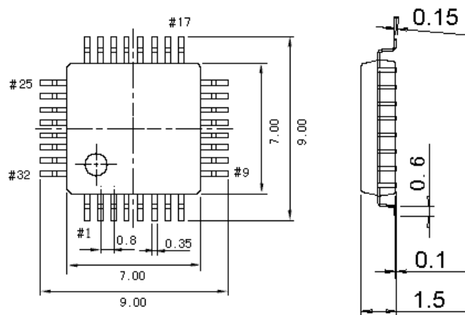
图 5-3 LQFP32 封装
