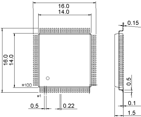
图 5-6 LQFP100 封装
